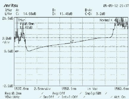
Диagr. 3 и 4. Кругизна характеристики (в принципе, оказалась нормальной для данного двухкаскадного EDFA)
