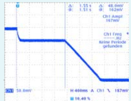
Диагр. 2. Очень долгое время выключения: 2,7 сек (!!!). Время детектирования исчезнувшего входного сигнала: 1,55 сек
