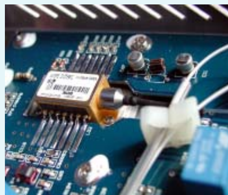
Фото 3.3. Вид сбоку на лазерный модуль: оригинальные электрические выводы более не существуют, и пайка произведена прямо к керамическому корпусу прибора
