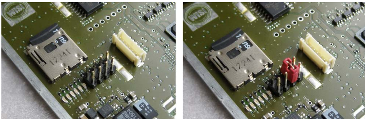
Рисунок 54. На левом снимке коммутатор в режиме «Неуправляемый простой коммутатор» (переключка J2 не установлена), на правом снимке коммутатор в режиме «Управляемый коммутатор с поддержкой VLAN» (переключка J2 установлена).
